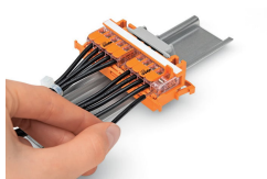
CAGE CLAMP®-Anschluss Leiter im Befestigungsadapter anschließen.
