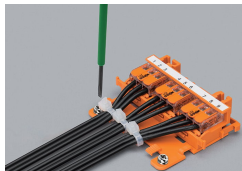
Liegende Schraubmontage mit Zugentlastungsplatte auf glatter Oberfläche
