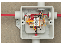
Anwendung im Klemmenkasten für Einbruchmeldeanlagen – Schraubbefestigung
