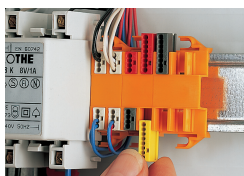
MICRO-Dosenklemme in den Adapter einschieben.
