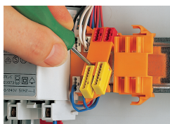
Befestigungsadapter aus dem Verband lösen.
