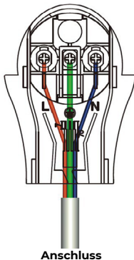
Anschluss
